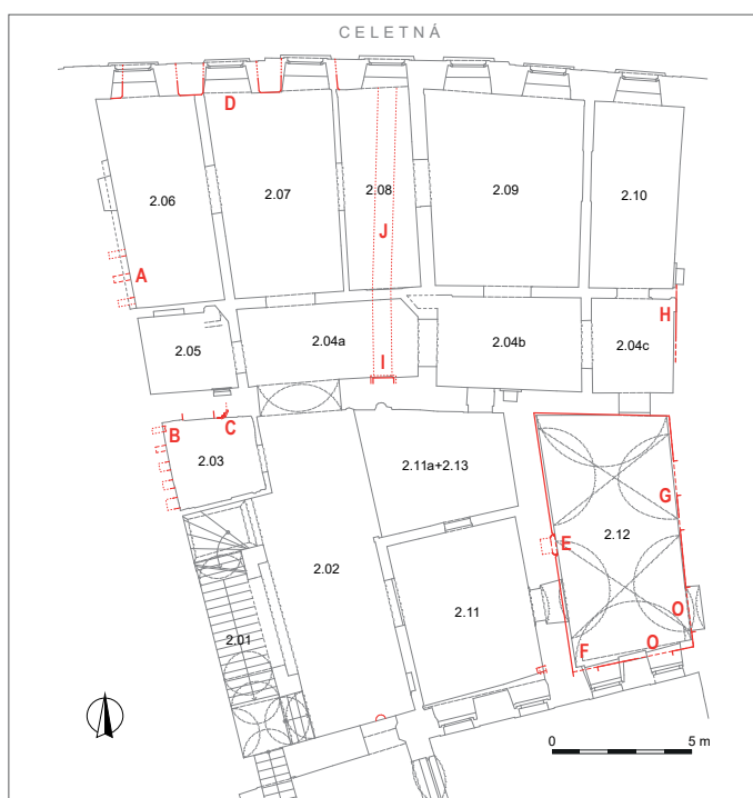
Obr. 11. Praha 1-Staré Město, čp. 553, Celetná 2, Sixtův dům. Půdorys 1. patra s vyznačením pozic vybraných nálezů. A – kapsy po stropních trámech, dokládající úroveň stropu nad přízemím raně gotického domu; B – kapsy po stropnicích z opravy po požáru, z jediného dochovaného trámového zhlaví byla získána datace 1301; C – bohatě profilovaná opuková portálová stojka; D – nález gotických meziokenních pilířů v průčelí z 1. čtvrtiny 14. století; E – gotická bohatě zdobená nika pod úrovní podlahy; F – pozice vstupu na převét (?), ještě v gotice zazděného; G – pozice původního vstupu do místnosti s jeho posunem k severu; H – nástěnná malba sv. Kryštofa; I – středověký opukový polopilíř; J – pozice středověké zdi, odbourané asi ve 30. letech 18. století; O – pozice zazděných oken (kresba A. Piskáčková, 2024).
