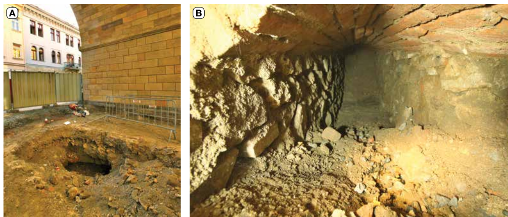
Obr. 14. Praha 8-Karlín, ppč. 871/34, Prvního pluku, stoka pod Negrelliho viaduktem. A – celková situace výkopu s porušenou klenbou stoky; pohled k jihovýchodu; B – vnitřek stoky – stěny z lomového kamene, cihelná klenba; pohled k jihovýchodu (foto A. Piskáčková, 2023).
