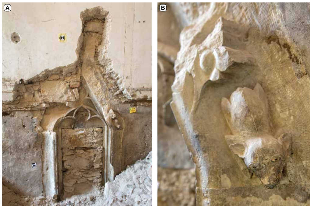
Obr. 10. Praha 1-Staré Město, čp. 553, Celetná 2, Sixtův dům. A – nika v západní zdi jihovýchodní místnosti 1. patra pod úrovní nynější podlahy, nalezená po vybrání násypu nad klenbou přízemí; B – dochované zvířátko, snad netopýr, na pravé straně niky (foto P. Havlík, 2021).
