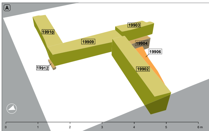
Obr. 21. Praha 1, Hradčanské nám. čp. 185/IV, sonda IX. 3D model zděných konstrukcí zástavby vrcholně středověké (před rokem cca 1370 – oranžové) a následné zástavby před požárem roku 1541 (základové zdivo hnědé, nadzemní zdivo zelené). A – pohled od severozápadu; B – pohled od jihu (podklady od firmy GEO-CZ z roku 2003 upravil F. Adámek, 2024).
