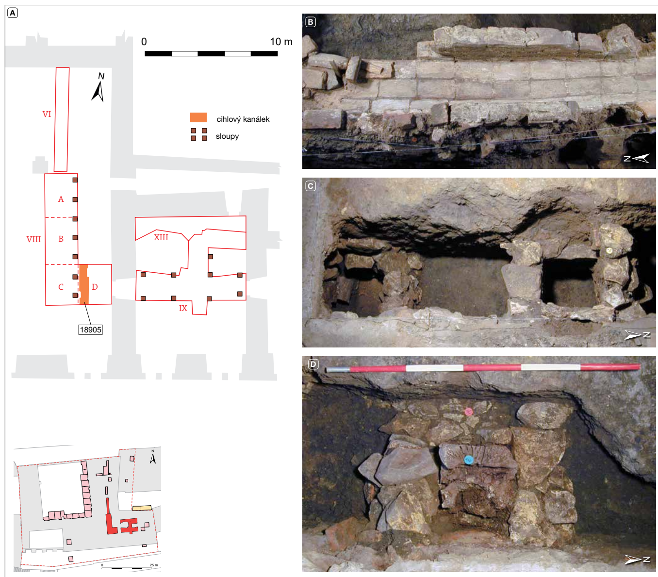
Obr. 55. Praha 1, Hradčanské nám. čp. 185/IV, sonda VIII. Koňské stáje. A – schematizovaný plán s relikty sloupů vymezujících jednotlivá stání pro koně; B – cihlový odtokový kanálek/žlábek (sektor VIII-D); C – kamenná konstrukce kolem původně dřevěných kúlů (VIII-B); D – detail dřevěného sloupu s kamennou konstrukcí v sektoru VIII-C (sestavil F. Adámek, 2024; foto G. Blažková, 2003).
