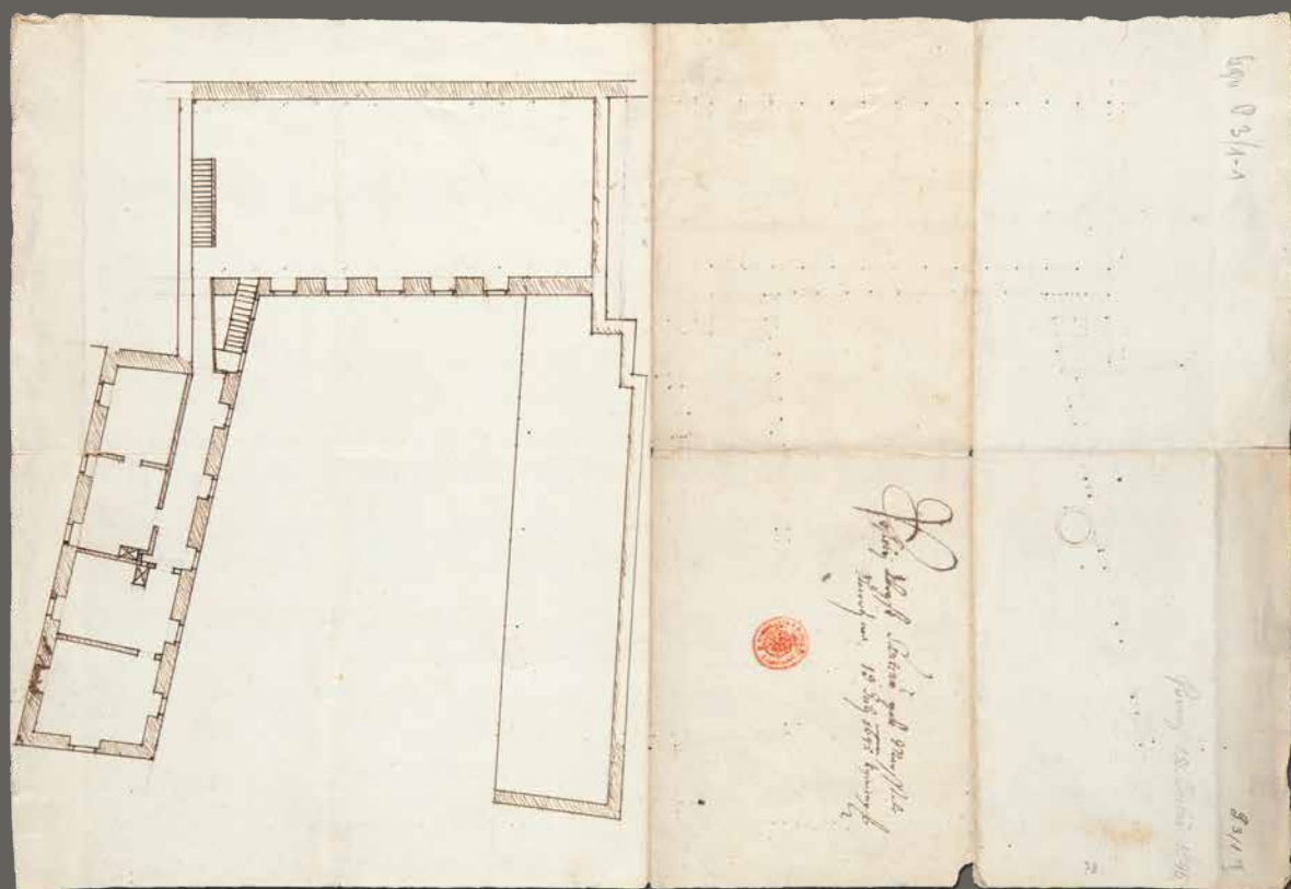
Obr. 12. Praha, Hrad, Jiřská čp. 7, rok 1645. Definitivní plánek půdorysu stavby maštali (Malého lobkovického domu čp. 7) v úrovni přízemí (A) a prvního patra (B), určený pro zednického mistra Santina de Bossi. Na rubu plánu je poznámka: „Poslední abrys Santinu jak maršale stavěti má, 19. Juli 1645 učiněný“ (Lobkowiczská knihovna a archiv, zámek Nelahozeves, Česká republika, LRRA, sign. P 3/1, fol. 78).
