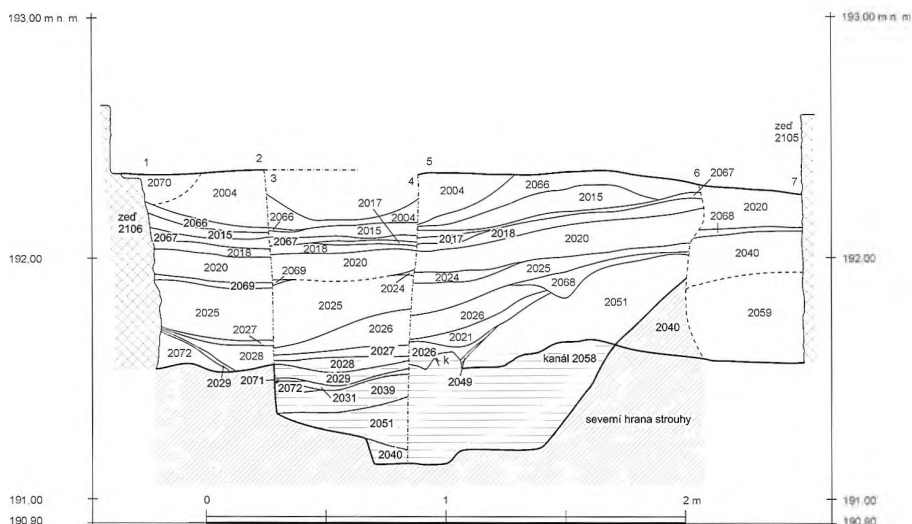
Obr. 1: Řez korytem odvodňovací strouhy.
