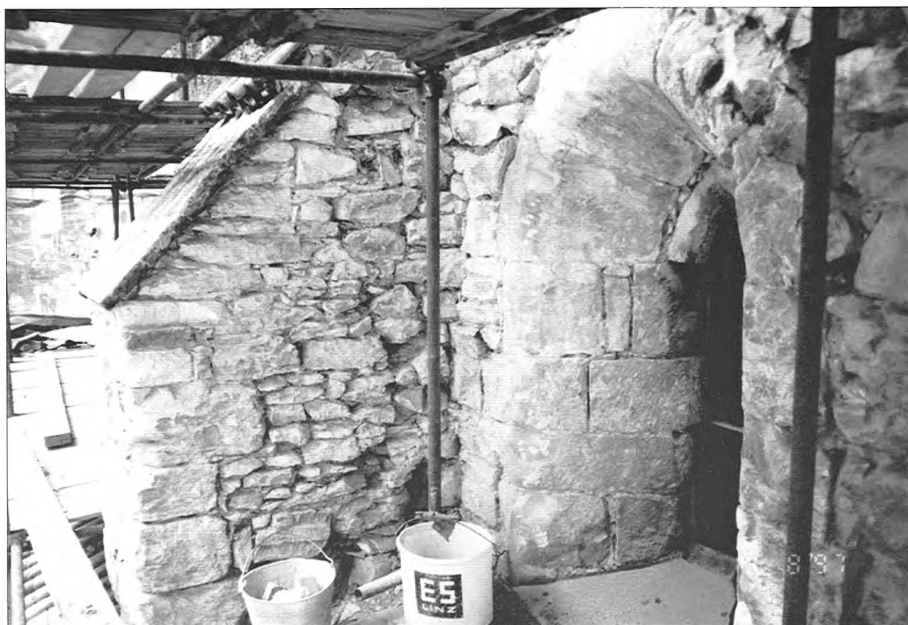
Obr. 8: Odhalené zdivo opěráku a ostění okna v jižní stěně Staronové synagogy (A. Pařík, 1998).
