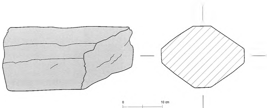
Obr. 6: Průřez okosených gotických sloupků nalezených pod podlahou bimy (21x16,5 cm), 1998.
