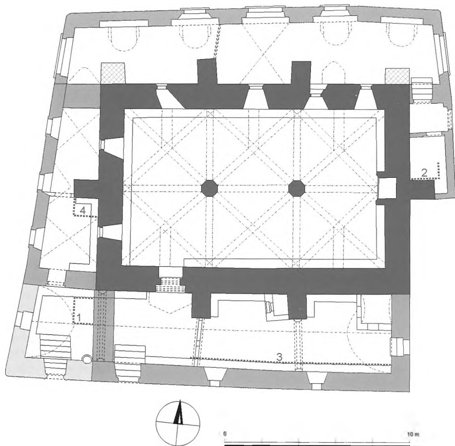
Obr. 1: Půdorys Staronové synagogy s vyznačením míst řezů historickými terény. Tmavočervená – jádro synagogy, červeně křížkovaně – základové statické zpevnění, světlejší červená – 2. gotická stavební fáze, světle červená – 3. gotická fáze, hnědá – barokní etapa z r. 1732. Kresba S. Matoušová.
