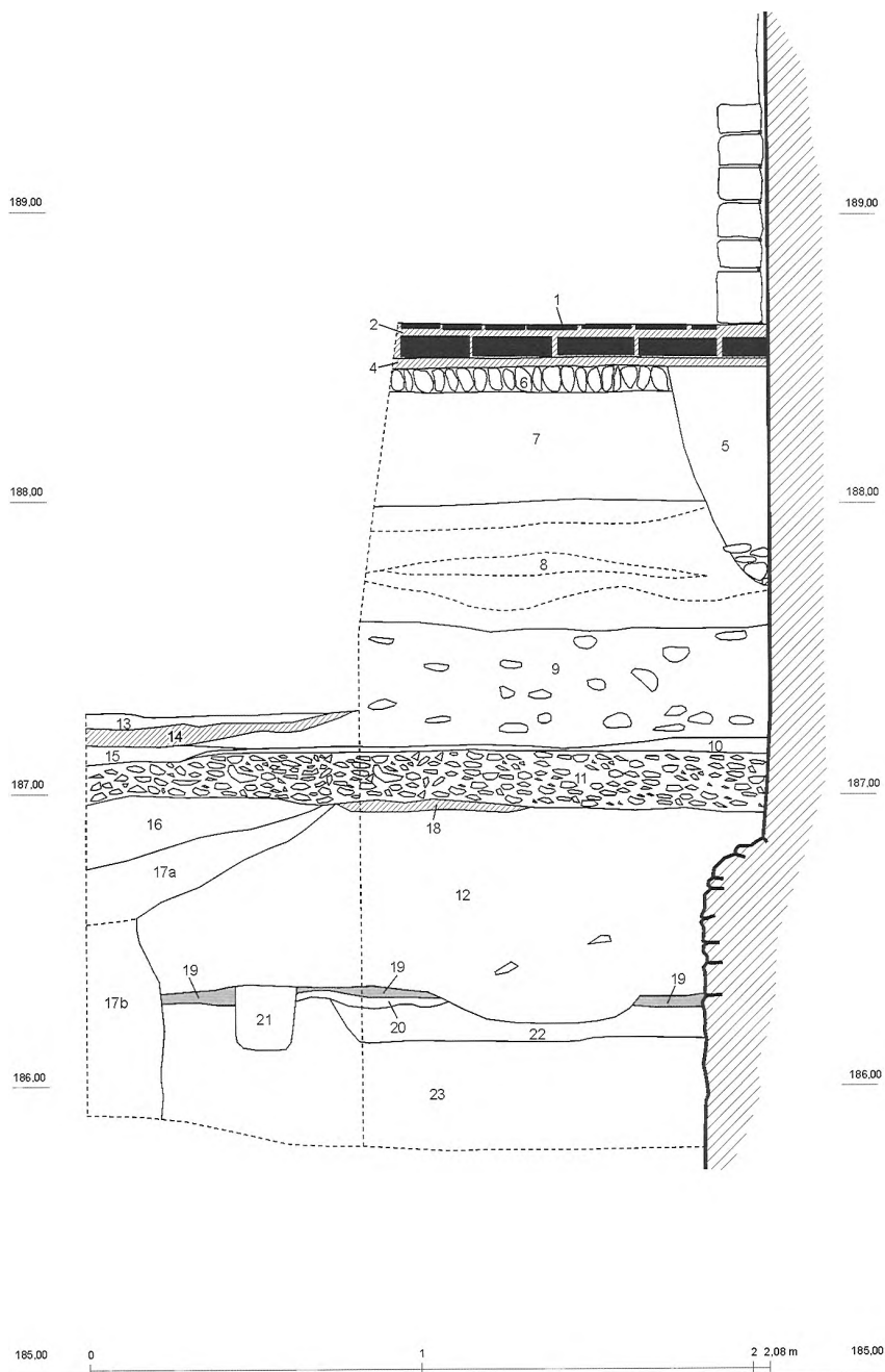
Obr. 2: Řez terény ve východním přístavku. Kresba Zd. Dragoun, S. Matoušová, M. Semerád.
