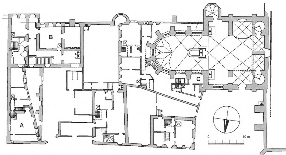
Obr. 3: Praha-Hrad, čp. 2/býv. tereziánský Ústav šlechticů. Plán zaniklé zástavby v západní části areálu Ústavu šlechticů asi z roku 1732. V ploše domu Jiljí de Roye (A) a domu děkana (B) byla nalezena zdíva, která nelze ztotožnit se zdívou na plánu. U „příbytku kaplanova“ (C) je shoda bezproblémová.
