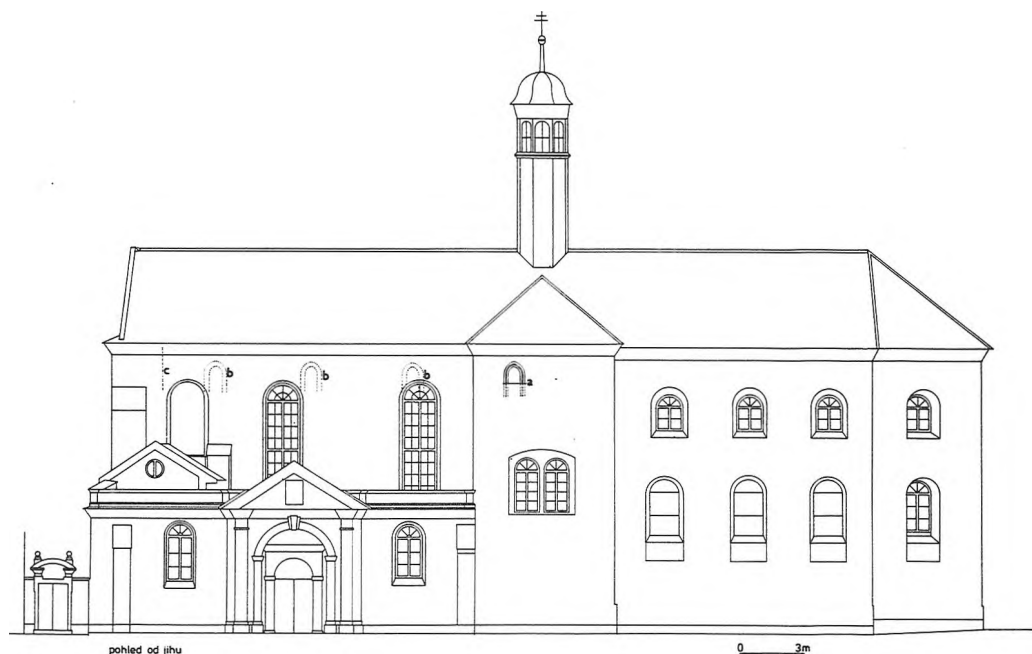
Jižní fasáda kostela sv. Jakuba, výsledky průzkumu: a — dochované gotické okno kryté transeptem, b — stopy zazděných gotických oken, c — spára oddělující gotické cihelné zdivo od pozdější stavby. (Zaměření a kresba J. Mourek)
