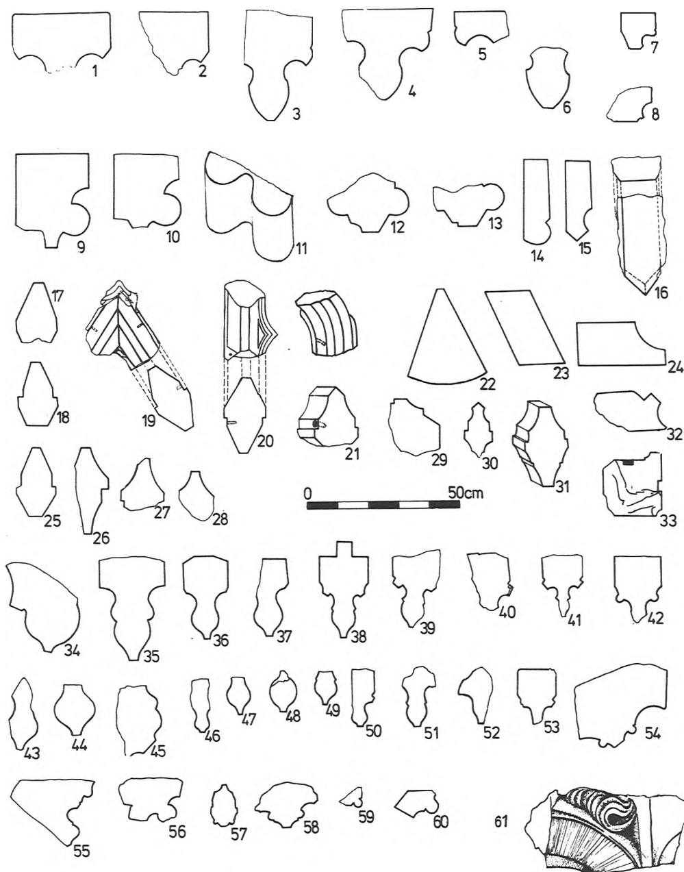
Přehled zlomků architektonických článků nalezených v letech 1976 — 1989 na Zbraslavi (o = opuka, p = pískovec, c = cihelná tvarovka): 1 p, 2 p, 3 p, 4 p, 5 p, 6 p, 7 o, 8 p, 9 c, 10 c, 11 o, 12 p, 13 p, 14 c, 15 c, 16 p, 17 c, 18 p, 19 p, 20 p, 21 p, 22 c, 23 c, 24 c, 25 p, 26 o, 27 o, 28 o, 29 p, 30 o, 31 o, 32 o, 33 p, 34 p, 35 p, 36 p, 37 p, 38 c, 39 c, 40 o, 41 p, 42 p, 43 o, 44 p, 45 p, 46 o, 47 c, 48 o, 49 o, 50 o, 51 o, 52 p, 53 o, 54 p, 55 p, 56 p, 57 o, 58 o, 59 o, 60 o, 61 o. (Kresby J. Mourek, repro R. Maleček)
