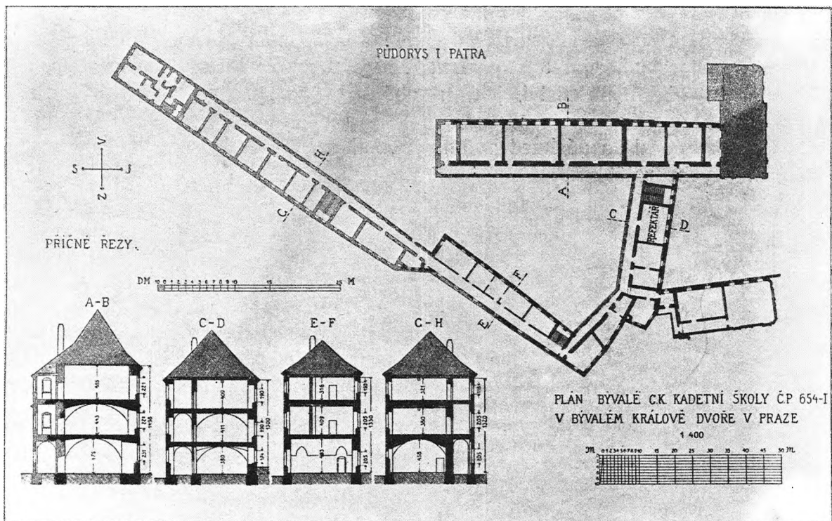
Zaměření Králova dvora – zaměření 1. patra a svislé řezy. (Repro R. Maleček)
