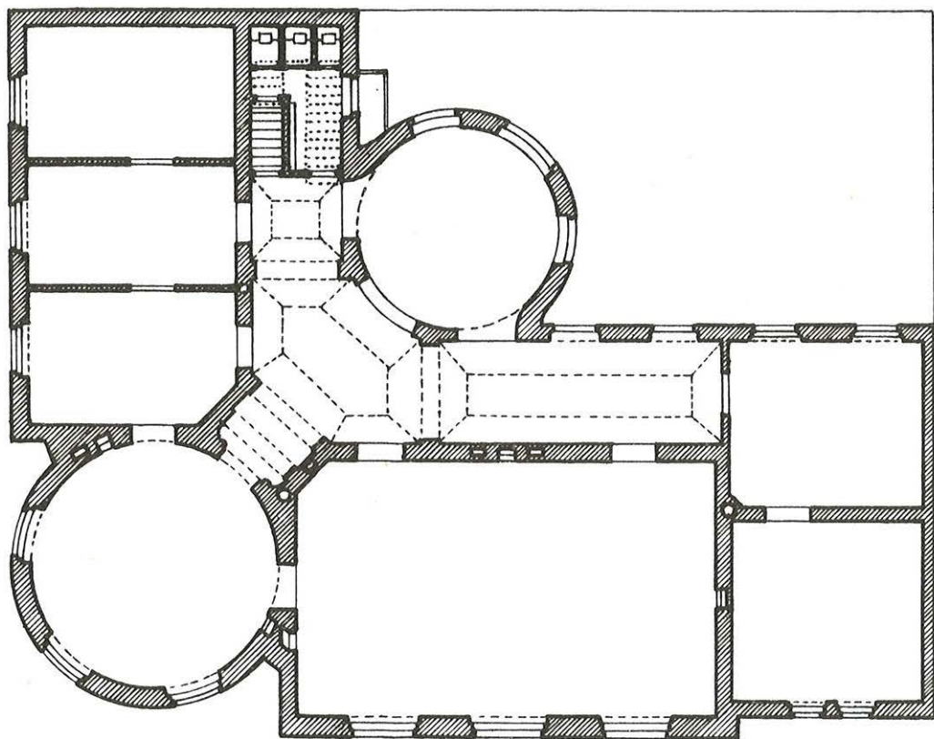
Návrh 2. patra žižkovské radnice z roku 1889.
