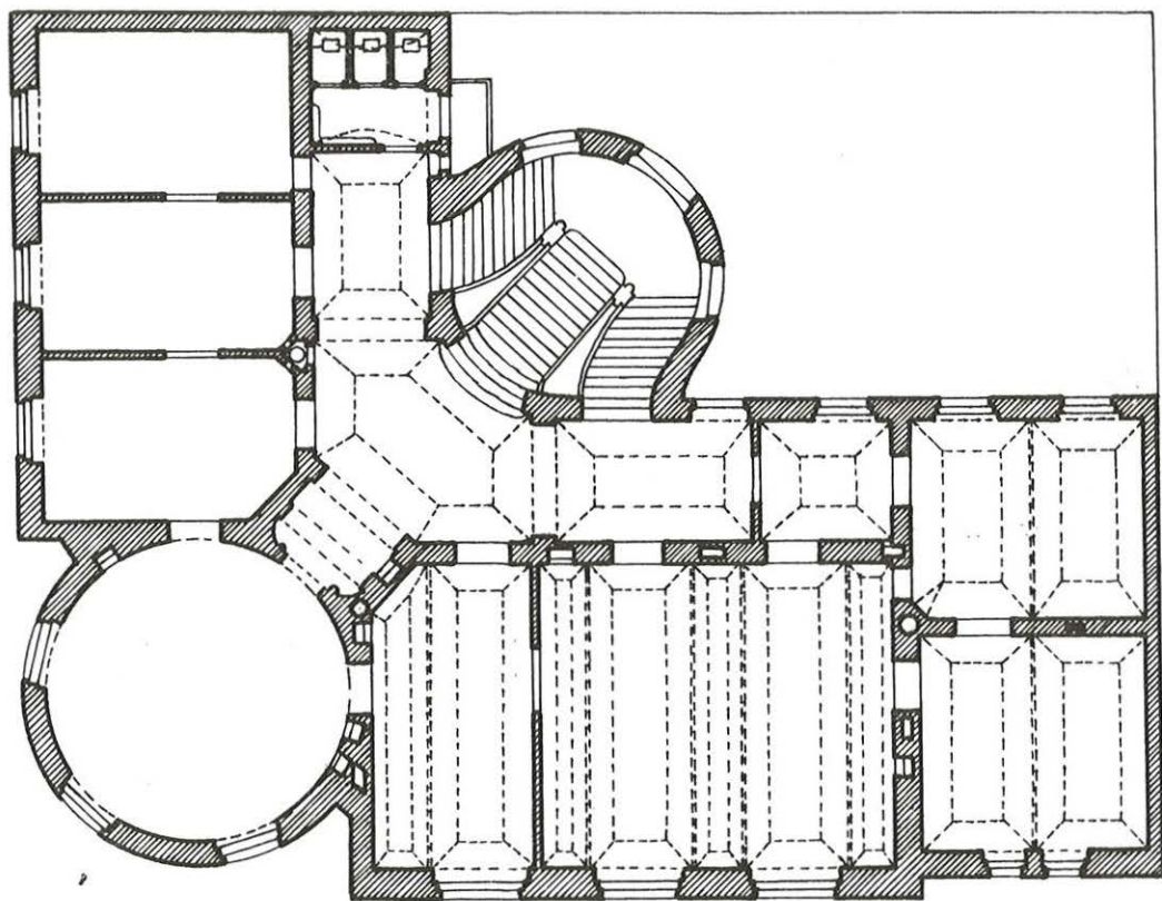
Návrh 1. patra žižkovské radnice z roku 1889.
