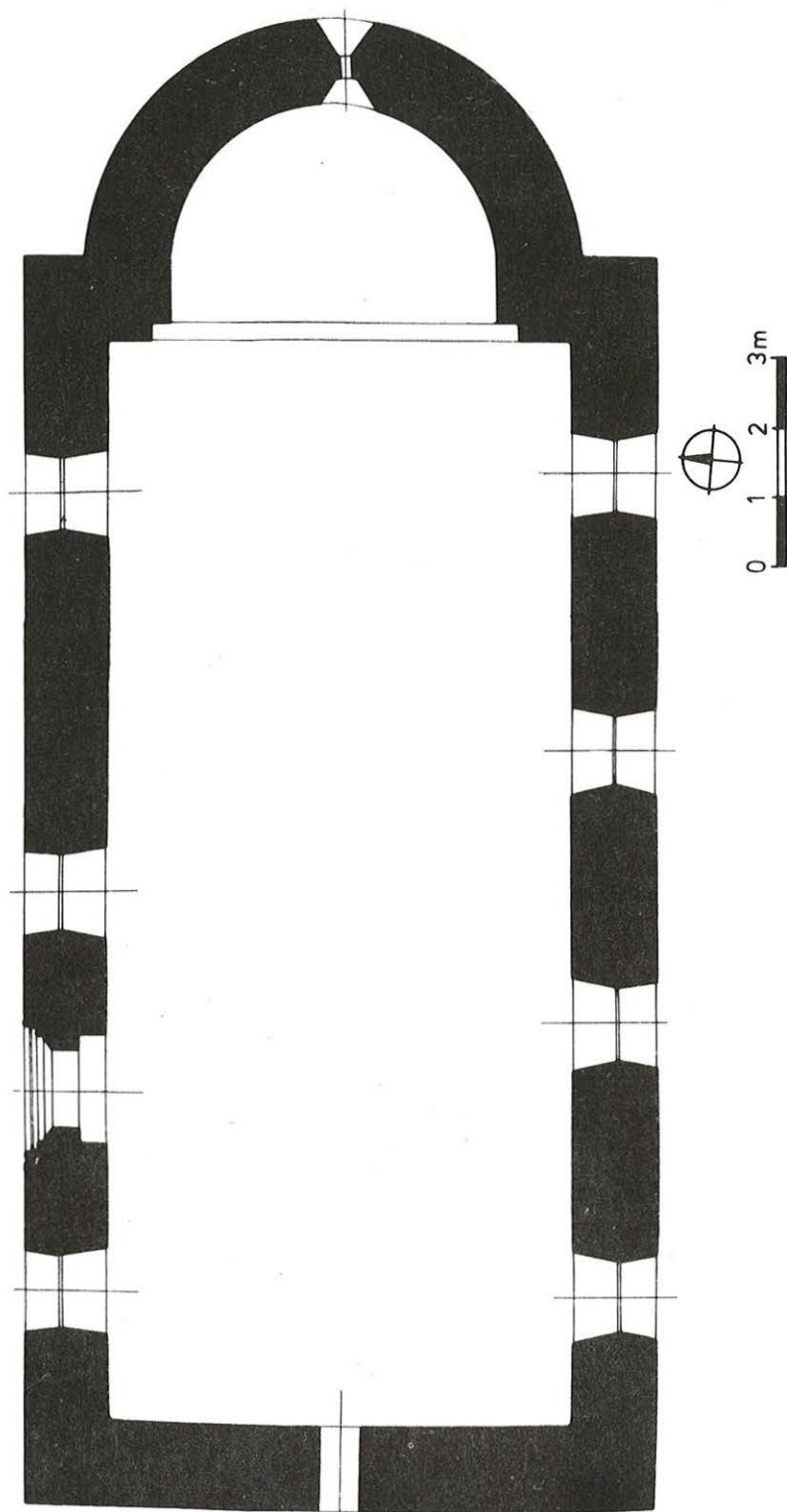
Rekonstruovaný půdorys kostela v době kolem poloviny 13. století.
