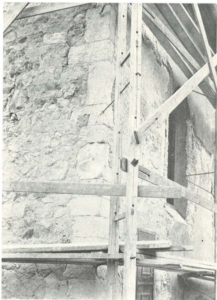
Jihozápadní nároží lodi kostela s opukovým nárožním armováním. V pozadí patrná západní část opukového ostění prvního původního okna od západu na jižní stěně lodi. Pohled od jihozápadu.
