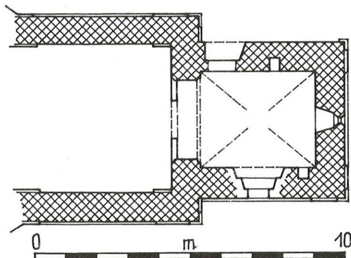
Kostel v Kunraticích. Půdorys gotické části dnešního kostela. Zaměření z roku 1987.
