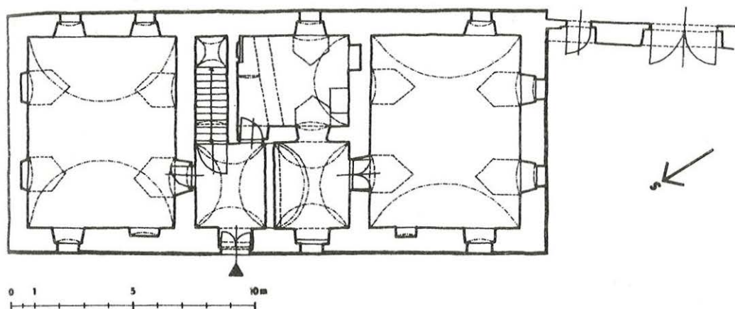
Půdorys přízemí domu usedlosti čp. 10 z doby nedlouho před rokem 1840 (podle zaměření SÚPPOP).
