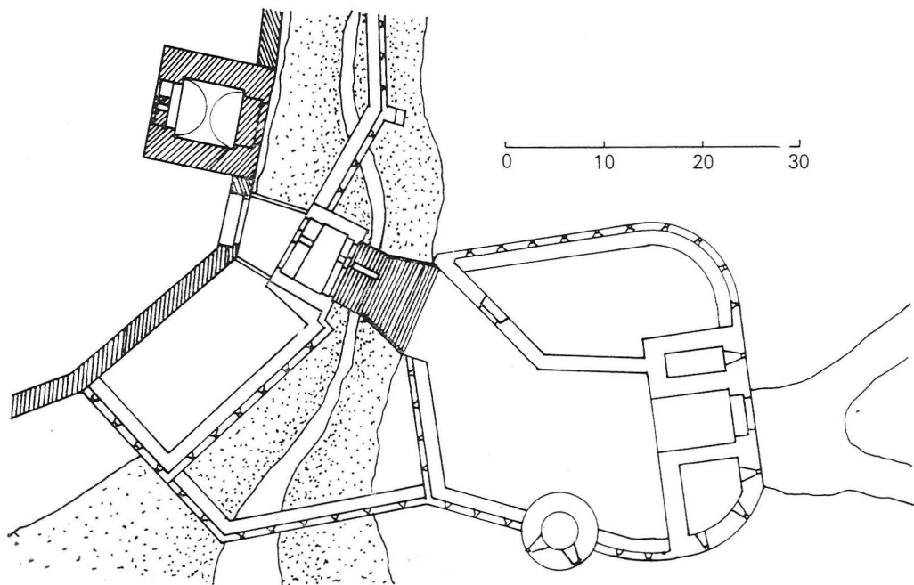
Východní předbraní Pražského hradu s barbakánem (R. Bied)
