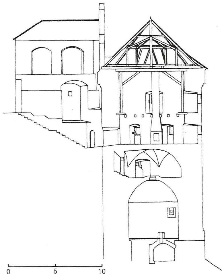
Severní část opevnění Pražského hradu, Daliborka – řez věží, pohled od západu (B. Ried) – podle D. Menclové
