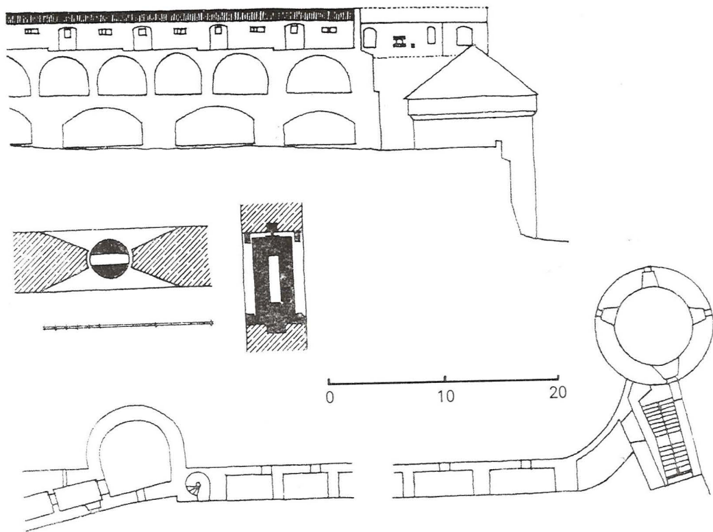
Severní část opevnění Pražského hradu, přízemí tzv. Bílé věže a Daliborky se slepými arkádami; půdorys a řez střílnou s otočným dřevěným bubnem; Daliborka a hradební zeď – vnitřek od jihu (B. Ried) – podle D. Menclové
