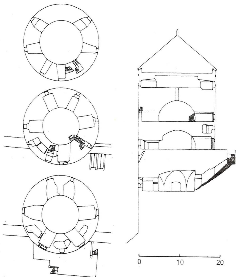
Severní část opevnění Pražského hradu, tzv. Mihulka – půdorys přízemí, 1. a 2. patra a příčný řez (B. Ried) – podle D. Menclové
