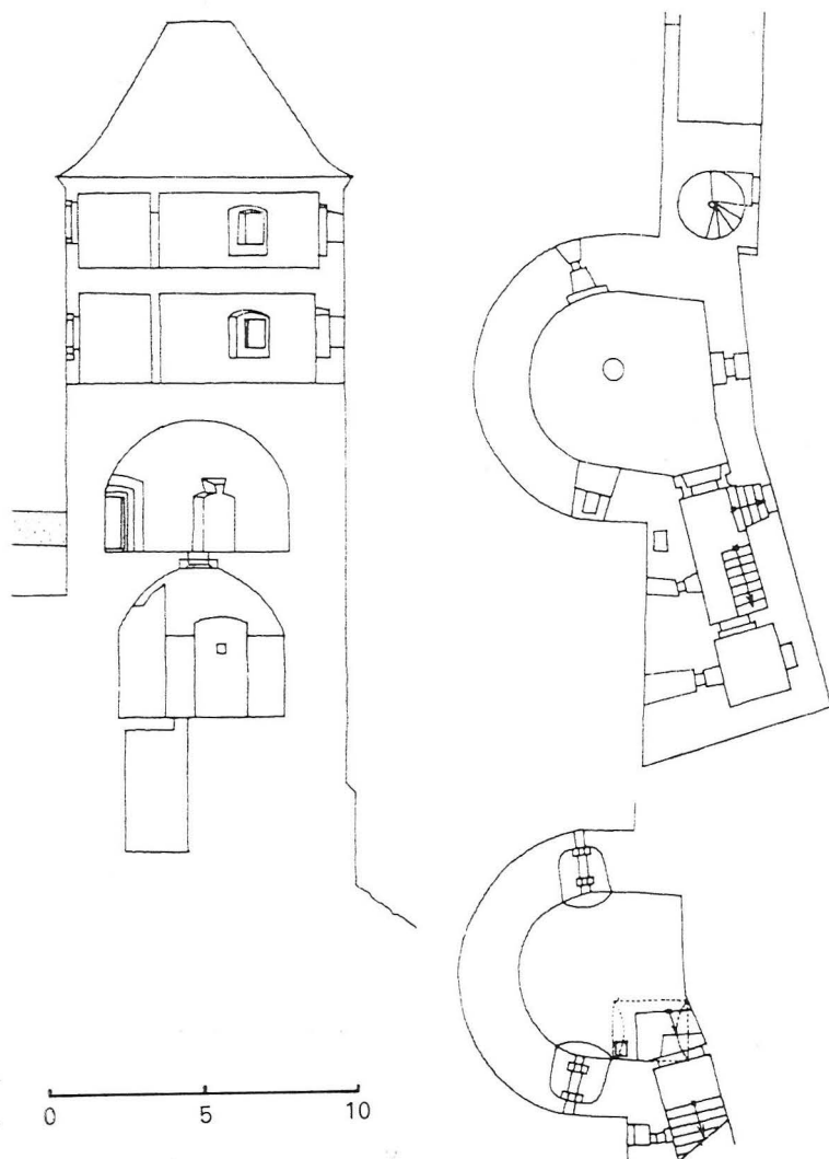
Severní část opevnění Pražského hradu, tzv. Bílá věž – půdorys suterénu a přízemí a příčný řez (B. Ried) – podle D. Menclové
