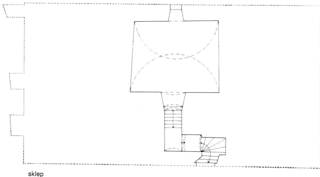
Čp. 7 – Benice, Praha 10 – zaměření suterénu
