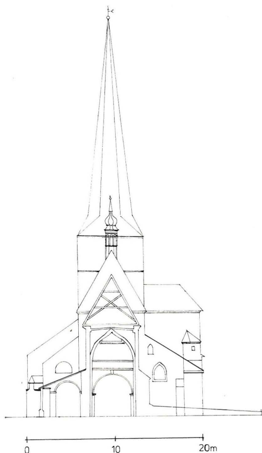
Kostel P. Marie Na louži, řez ve směru S–J. Podle kopie bouracích plánů
