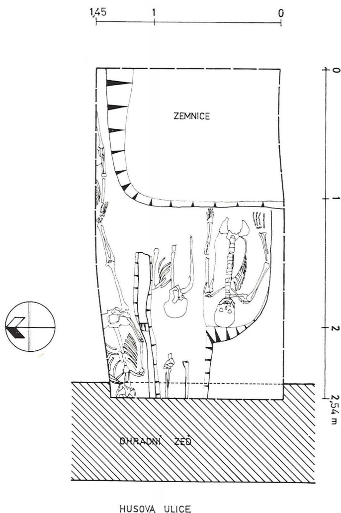
Půdorysný plán sondy archeologického výzkumu. Horizont hrobů porušen výkopem pro zemnici
