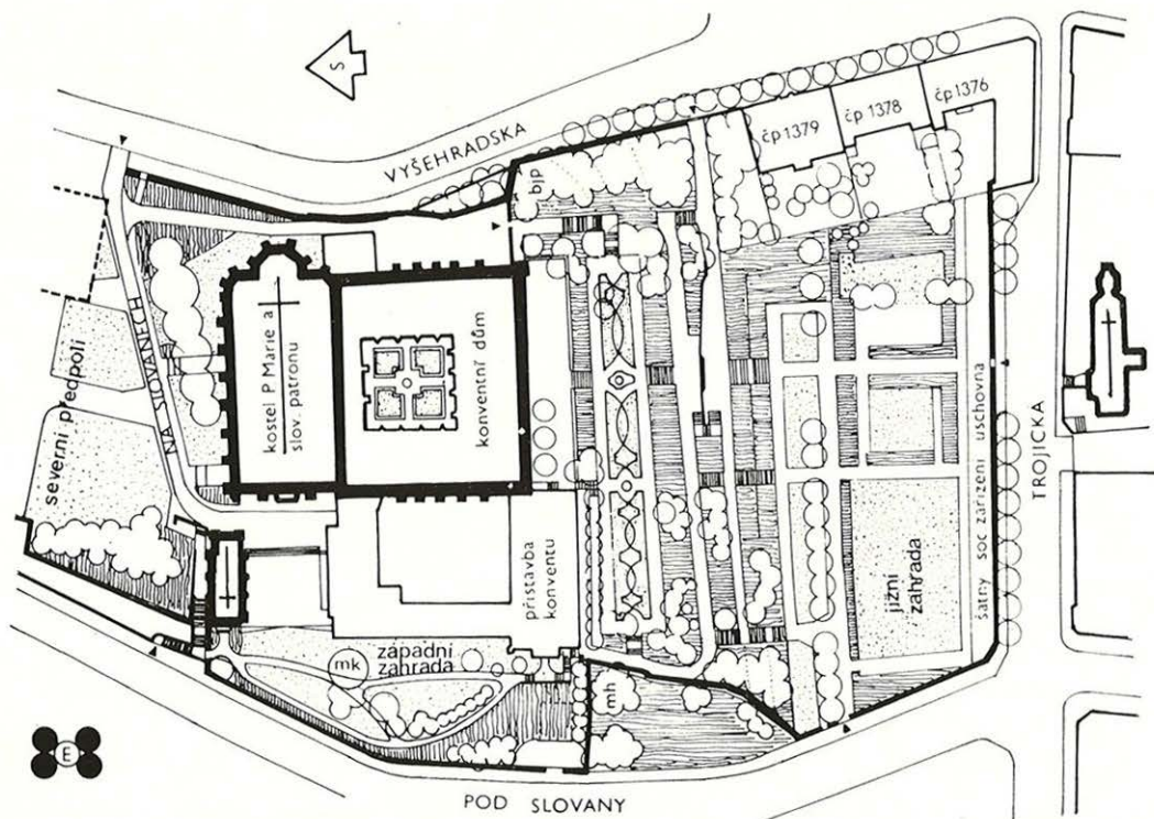
Návrh úpravy emauzských zahrad podle situace ze studie B. Pavelkové, M. Krumla a M. Haase (kresba J. Pavelka)
