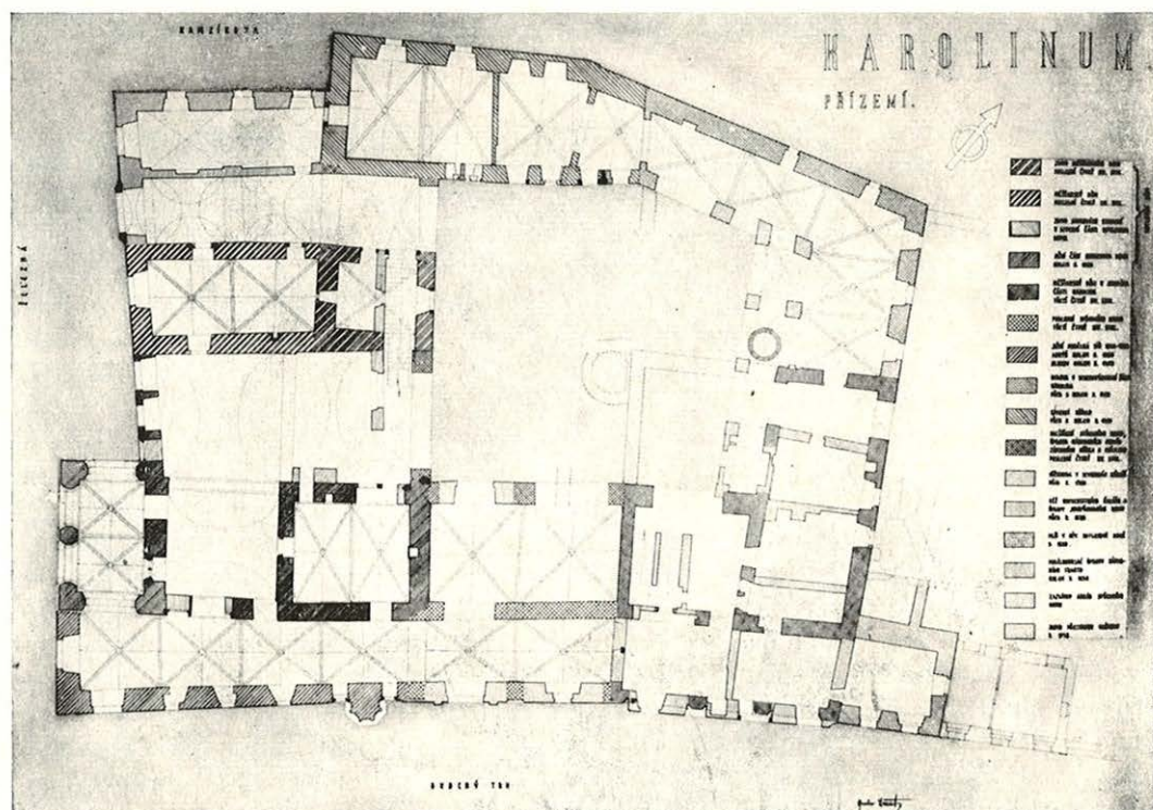
Karolinum – půdorys přízemí (kresba M. Ernest, reprodukce Z. Helfert)
