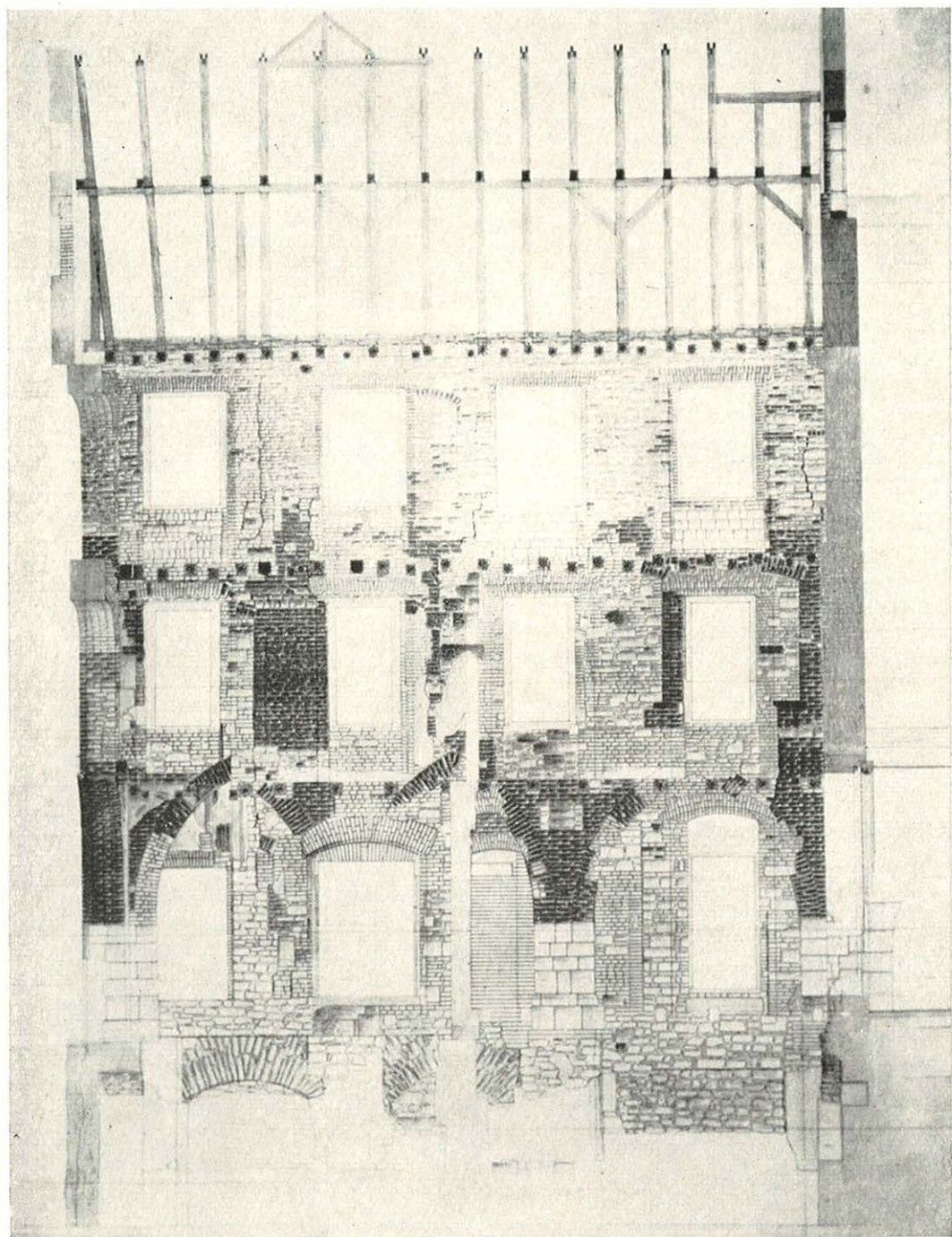
Zachované části gotických arkád Karolina (kresba M. Ernest, reprodukce J. Janáková)
