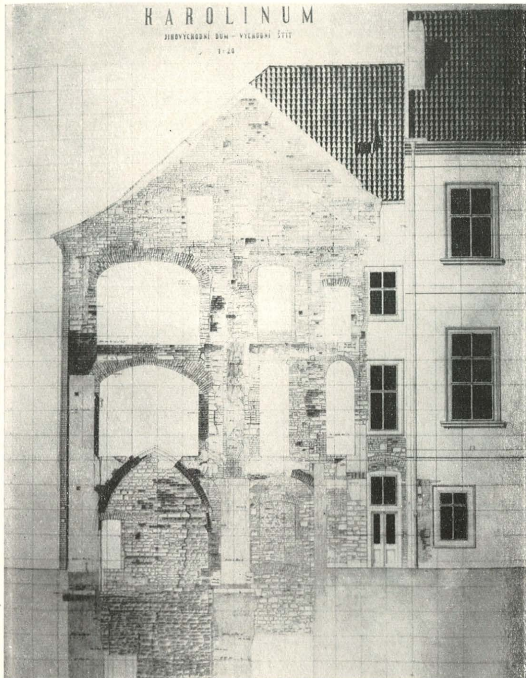
Karolinum, východní štít (kresba M. Ernest, reprodukce Z. Helfert)
