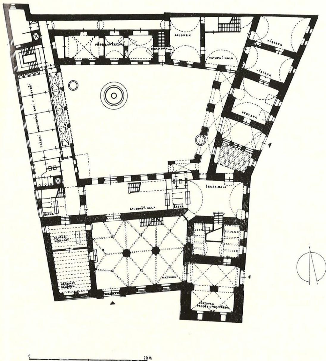
Studie na úpravu Novoměstské radnice – přízemí (kresba arch. F. Kašíčka, reprodukce K. Kibic)
