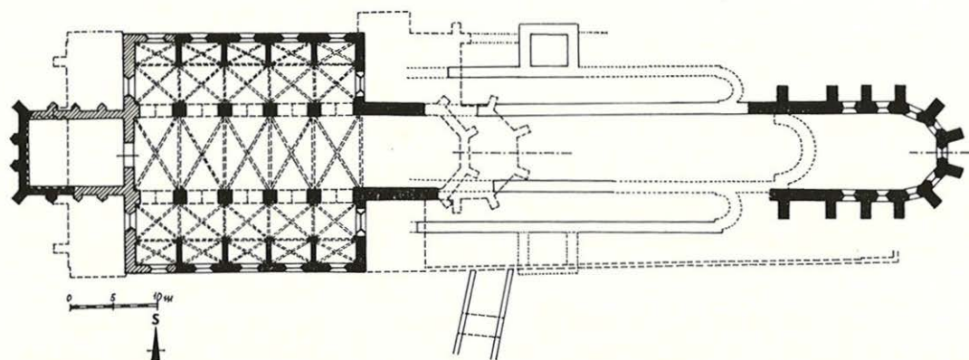
Pracovní rekonstrukce půdorysu kapitulního kostela sv. Petra a Pavla na Vyšehradě ve 14. století – černě označeny gotické doložené konstrukce, šrafovaně předpokládané, bíle ponechány nalezené a předpokládané základy románské baziliky, věží a mostu (kresba F. Kašíčka)
