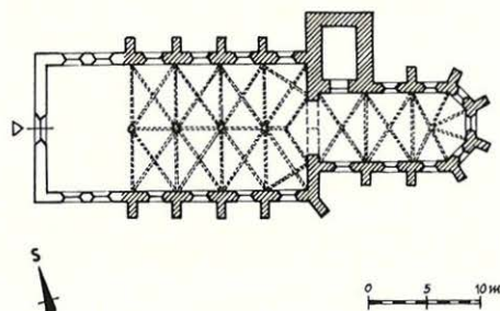
Rekonstrukce jižního průčelí a půdorysu kostela Pokory Panny Marie (sv. Alžběty) v Podvyšehradě ve 14. století (kresba F. Kašička)
