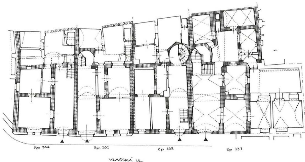
Půdorys přízemí skupiny domů čp. 331—334/III, ve Vlašské ulici na Malé Straně. Křížkováním vyznačeno renesanční zdivo. Navrhli M. Heroutová a D. Líbal.
