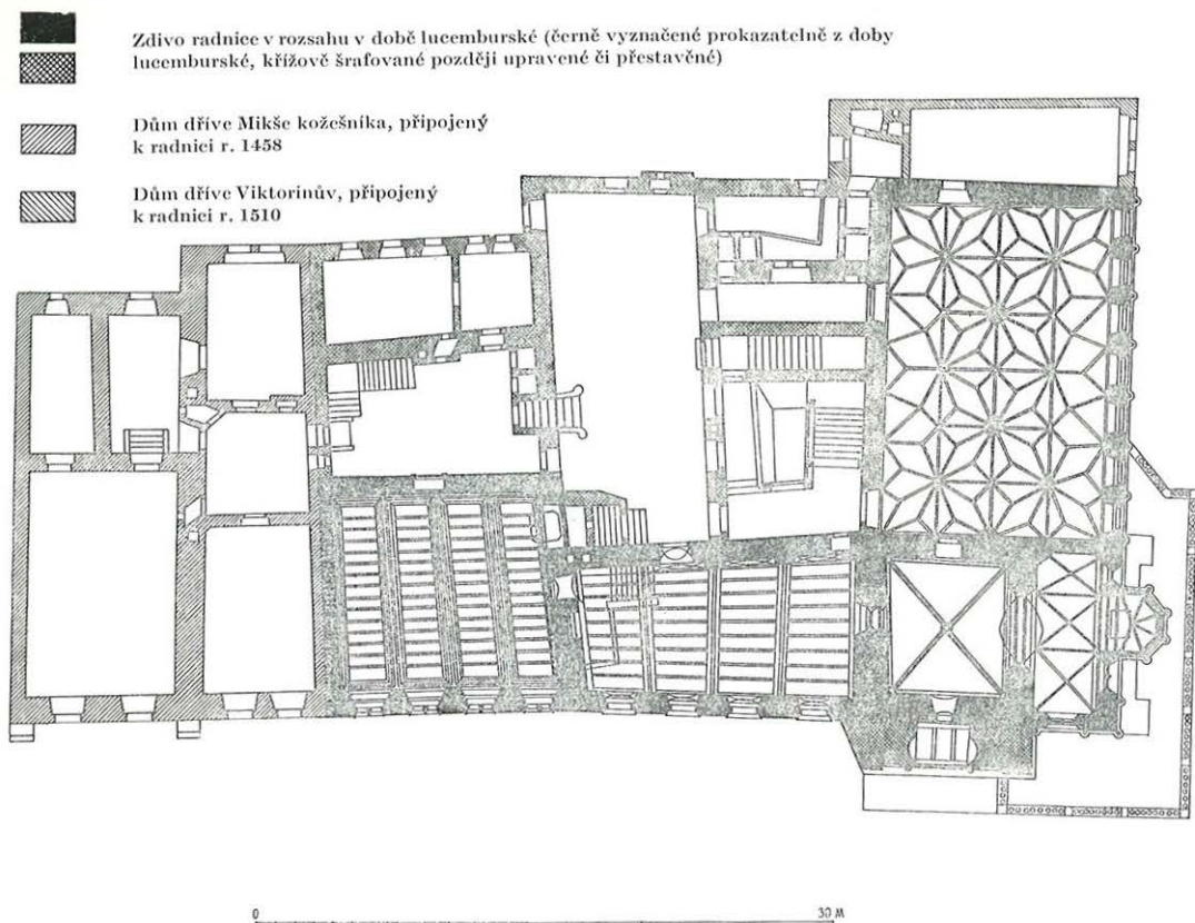
Původní rekonstrukce prvního a druhého patra (kresba K. Kibic)
