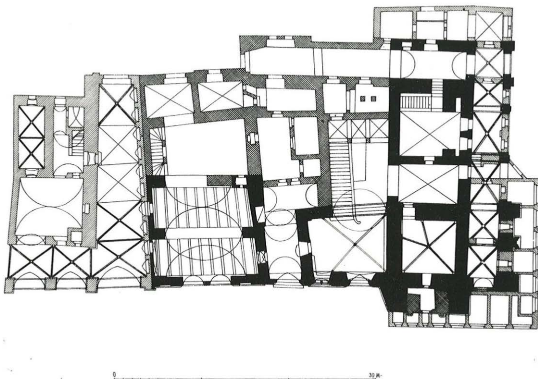
Rekonstrukce původního přízemí (kresba K. Kibic)
