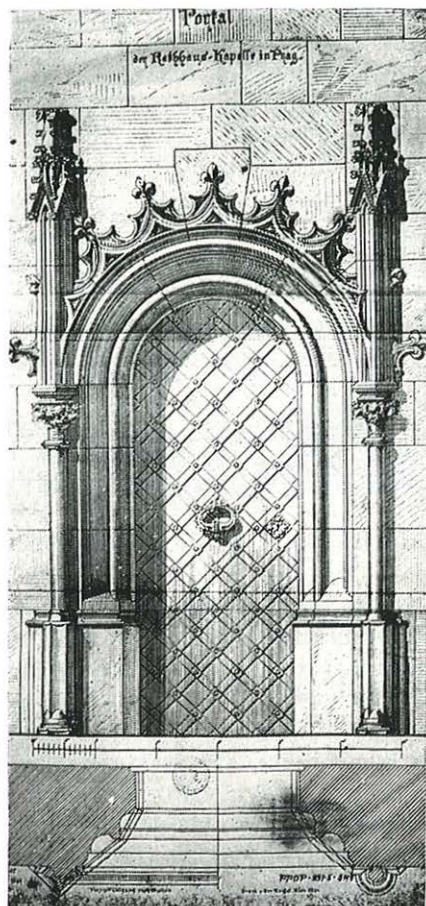
Nárys portálu ve věžní části kaple (reprod. K. Kibic)
