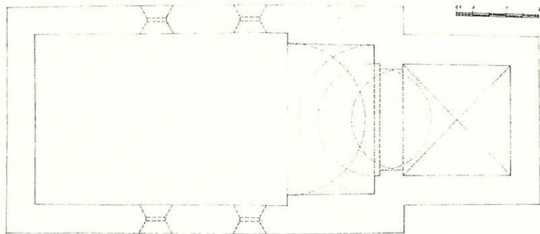
Kostel sv. Vavřince pod Petřínem na Újezdě, rekonstrukce románského stavu podle nálezů — půdorys (kolem poloviny 12. stol.).
