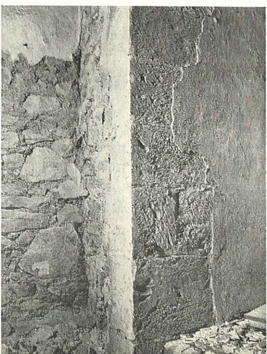
Býv. kostel sv. Vavřince pod Petřínem na Újezdě, oprávacování nárožních kvádrů při jižním rozšíření podvěžního zdiva, vlevo za nárožím zbytky osekaneho románského triumfálního oblouku (foto J. Janatková)
