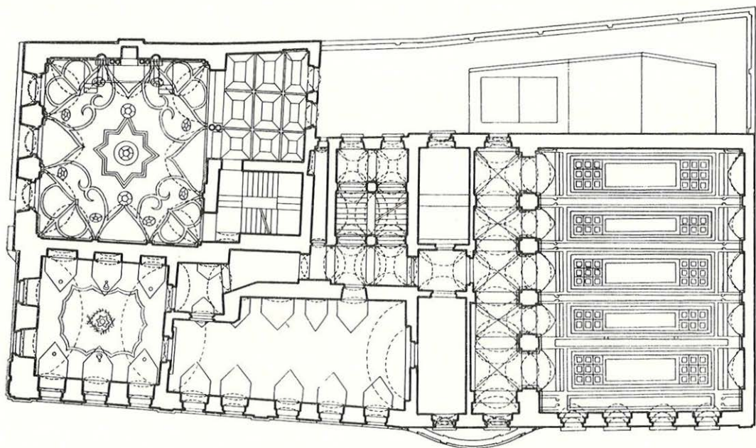
Půdorys 1. patra radnice, Vysoké synagogy a přístavby z r. 1908 — současný stav (zaměř. K. Kibic)
