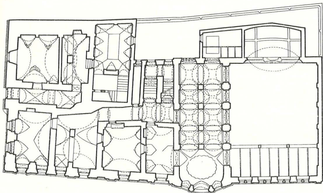
Půdorys přízemí radnice, Vysoké synagogy a přístavby z r. 1908 — současný stav (zaměř. K. Kibic)
