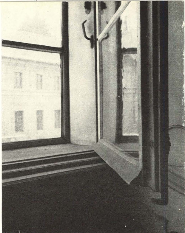
Arcibiskupský palác — 2. patro jižního průčelí — svodnice pro dešťovou vodu u vnitřního okna
