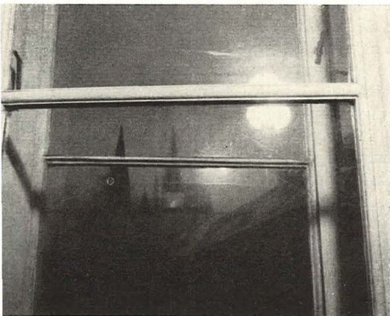
Arcibiskupský palác — příčníky vnějšího a vnitřního okna v 2. patře východního průčelí různost profilace
