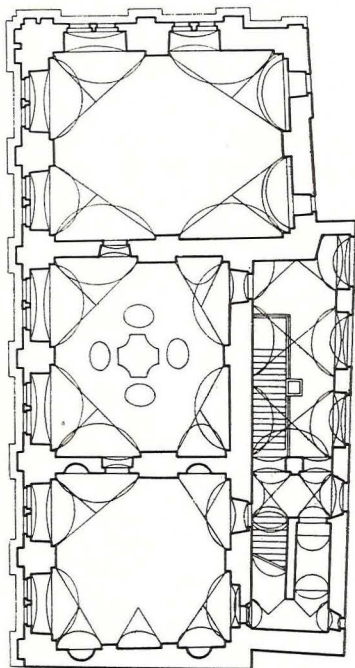
Půdorys 1. patra Malostranské radnice
