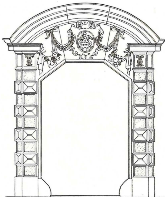
Portál v radničním vestibulu
