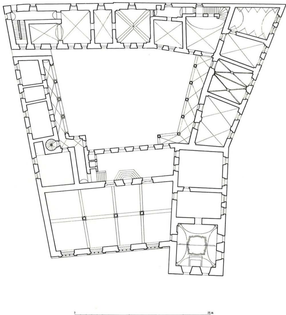
Dispozice 1. patra Novoměstské radnice. Rekonstrukce původního stavu. — Kresba: K. Kibic
