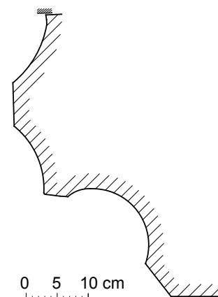
Obr. 8. Praha 1-Staré Město, čp. 1/1, Staroměstská radnice, věž. Profilace ostění okna v jižní fasádě (kresba L. Bartoš, 2017).
