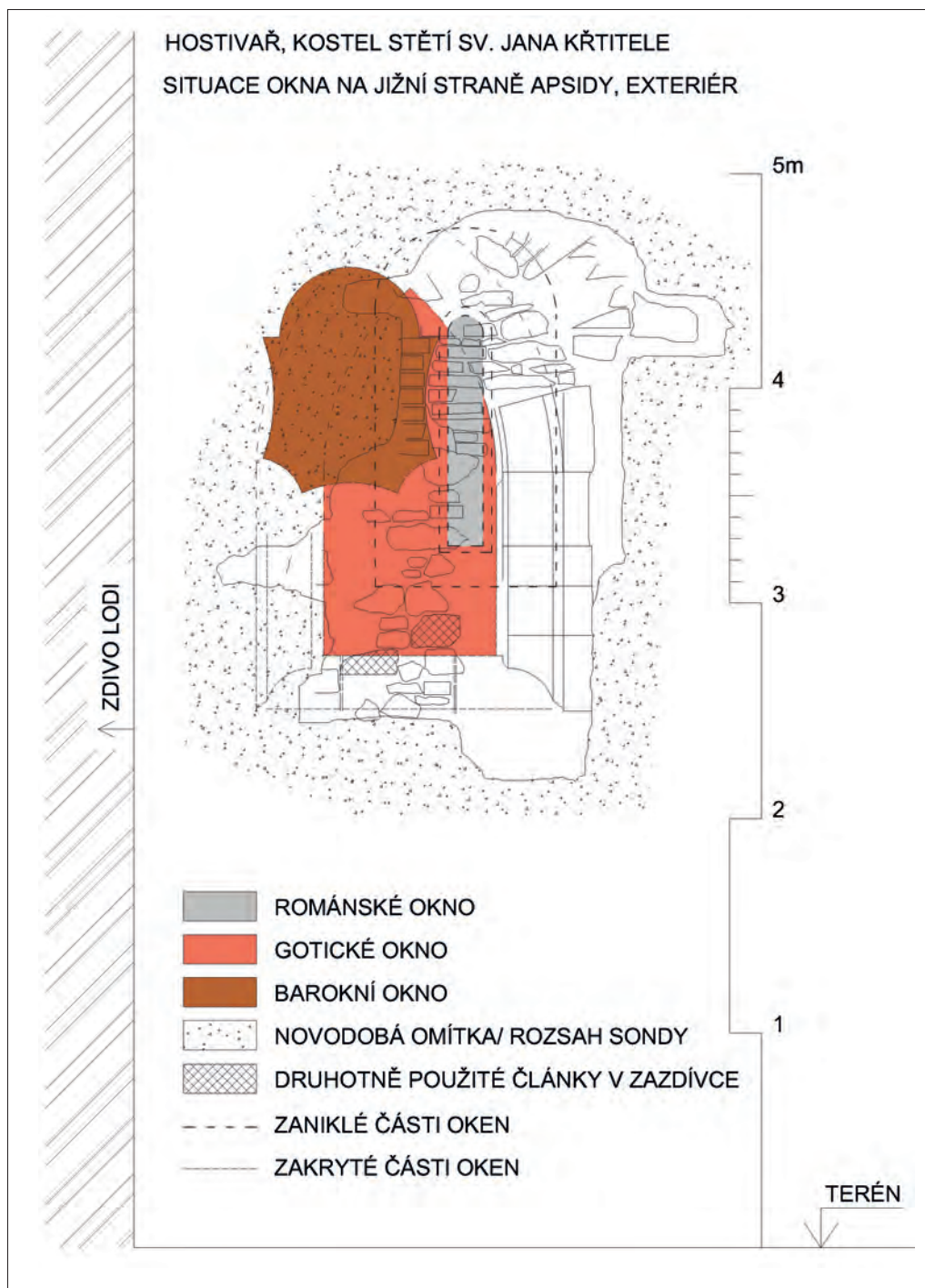
Obr. 7. Praha-Hostivař, kostel Stětí sv. Jana Křtitele. Jižní okno apsidy v pohledu z exteriéru. Srovnání polohy a velikosti okenního otvoru románského, gotického a barokního (L. Bartoš, 2010, 2014).
